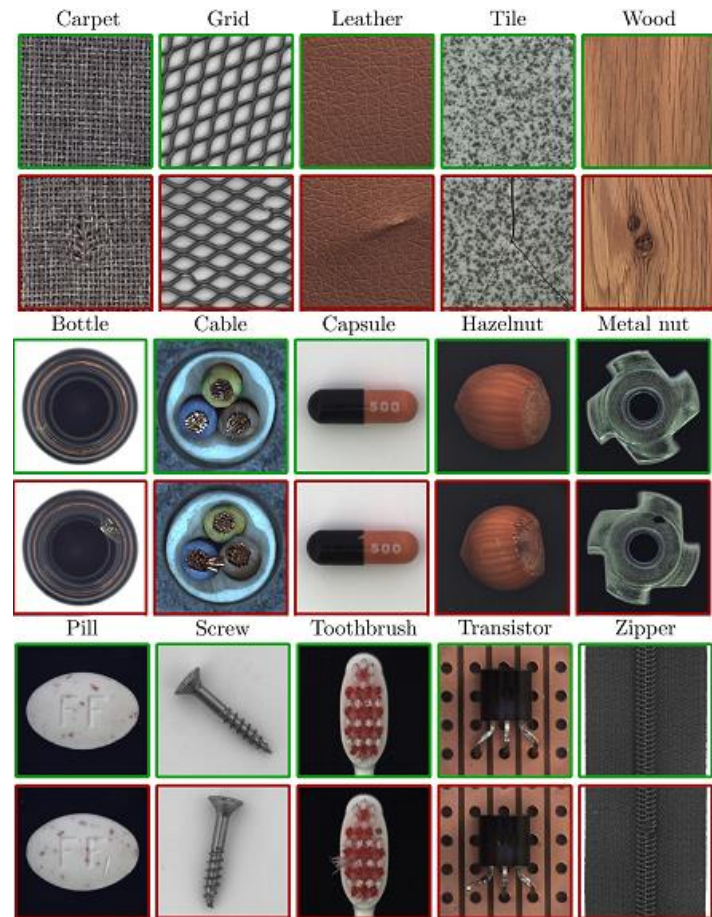
Fig. 6 MVTec Dataset
